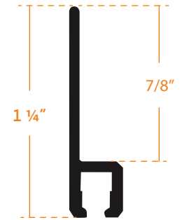
VISTA LATERAL Perfil Vertical.
